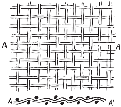
FIGURE 8.1. Plain weave (tafetán) . Top, top view; bottom, side view. (Redrawn from Mastache, "El Tejido en el México antiguo," Arqueología Mexicana, Edición especial 19 [2005]: 29.)
