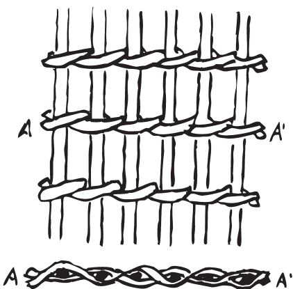
FIGURE 8.2. Joining (enlazado) . Top, top view; bottom, side view. (Redrawn from Mastache, “El Tejido en el México antiguo,” Arqueología Mexicana, Edición especial 19 [2005]: 30.)
